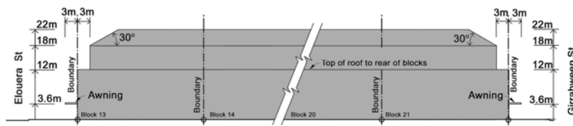
Elevation 2
